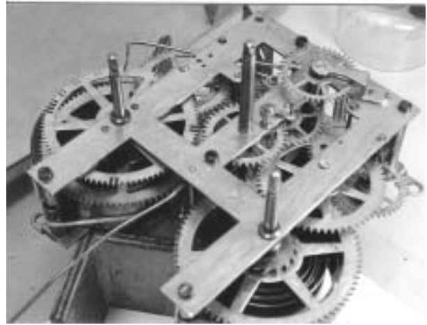
Amerikkalainen lyönnillisen kellon koneisto 1800-luvun loppupuolelta.
